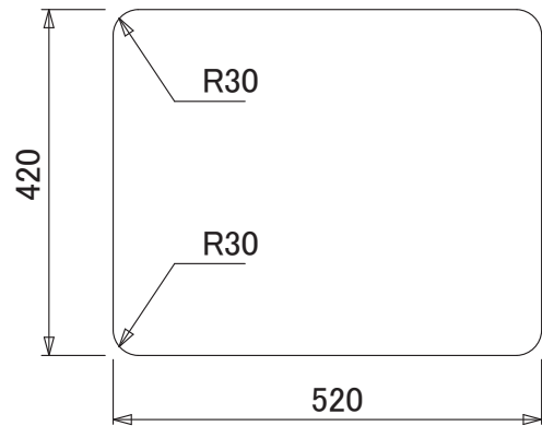
カウンター開口寸法
